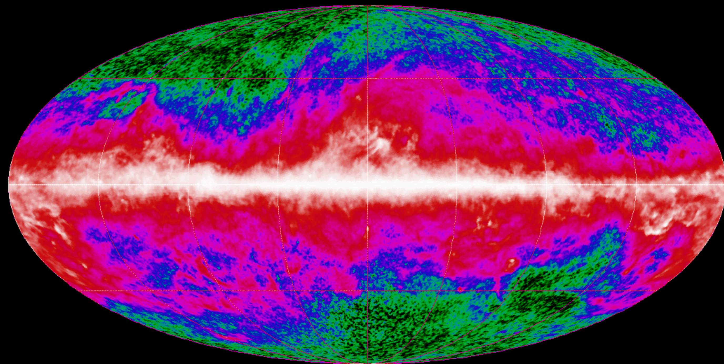
DIRBE 240 MICRONS, MJY/SR
