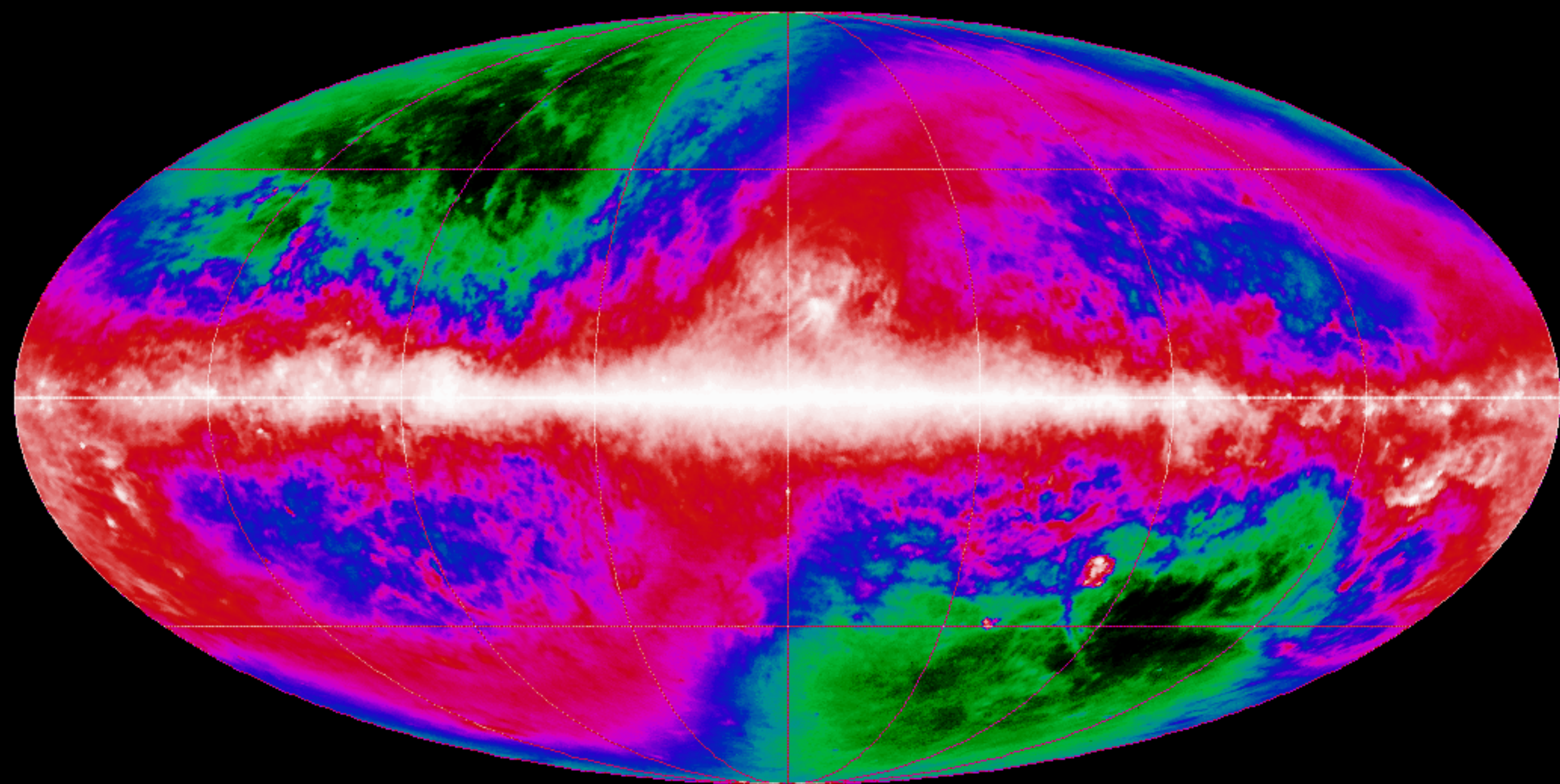
DIRBE 100 MICRONS, MJY/SR
