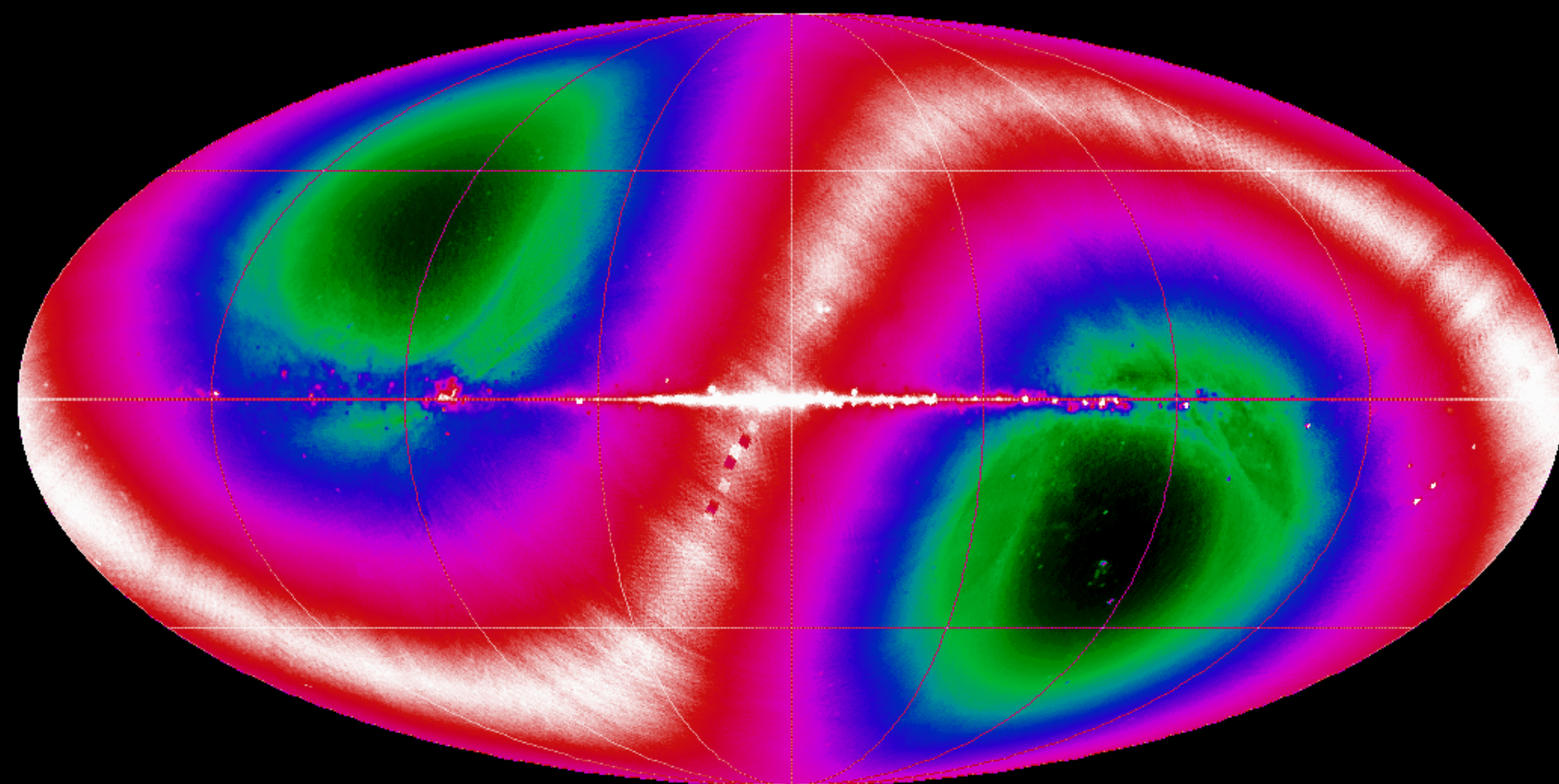
DIRBE 25 MICRONS, MJY/SR
